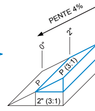
(B) COUPE
