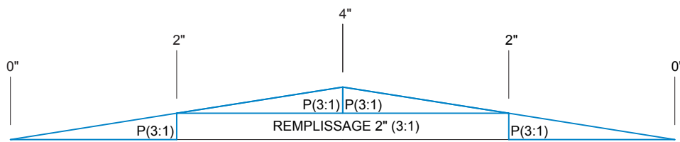
(A) COUPE
