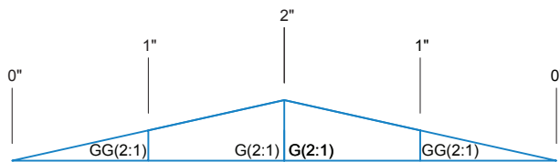
(A) COUPE
