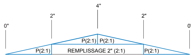
(A) COUPE
